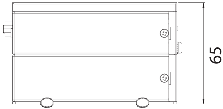
Рисунок 4. Габаритные и монтажные размеры системного блока RTU-327L и RTU-327LV
